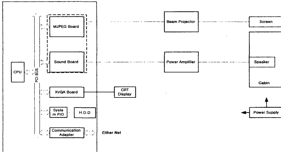
( 그림 3. A/V cabinet )
