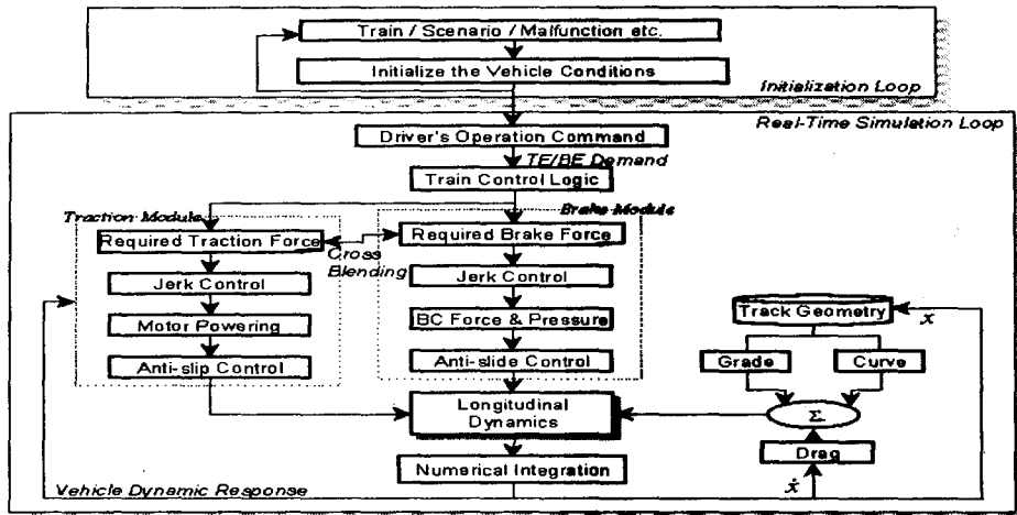
( 그림 6 : 모델링 구현 Block Diagram )
