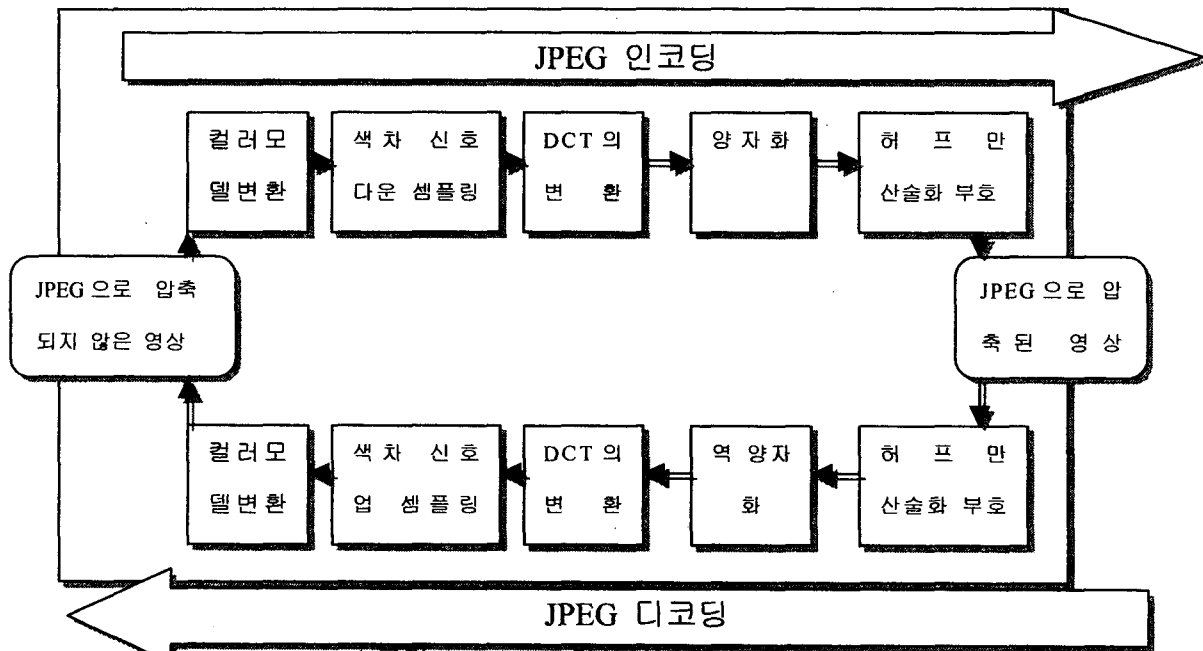
( 그림 2: JPEG 영상 시스템 )
