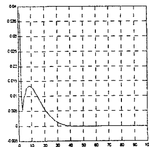
그림 2. 반향경로의 충격응답 Fig 2. Impulse Response of Echo Path
