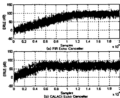
그림 5. FIR과 CALAOI 반향 제거기의 성능 비교 Fig 5. Performance Evaluation of FIR and CALAOI Echo Canceller
