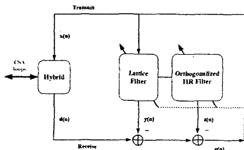
그림 3. 제안된 반향 제거기의 블록도 Fig 3. Block Diagram of Proposed Echo Canceller
