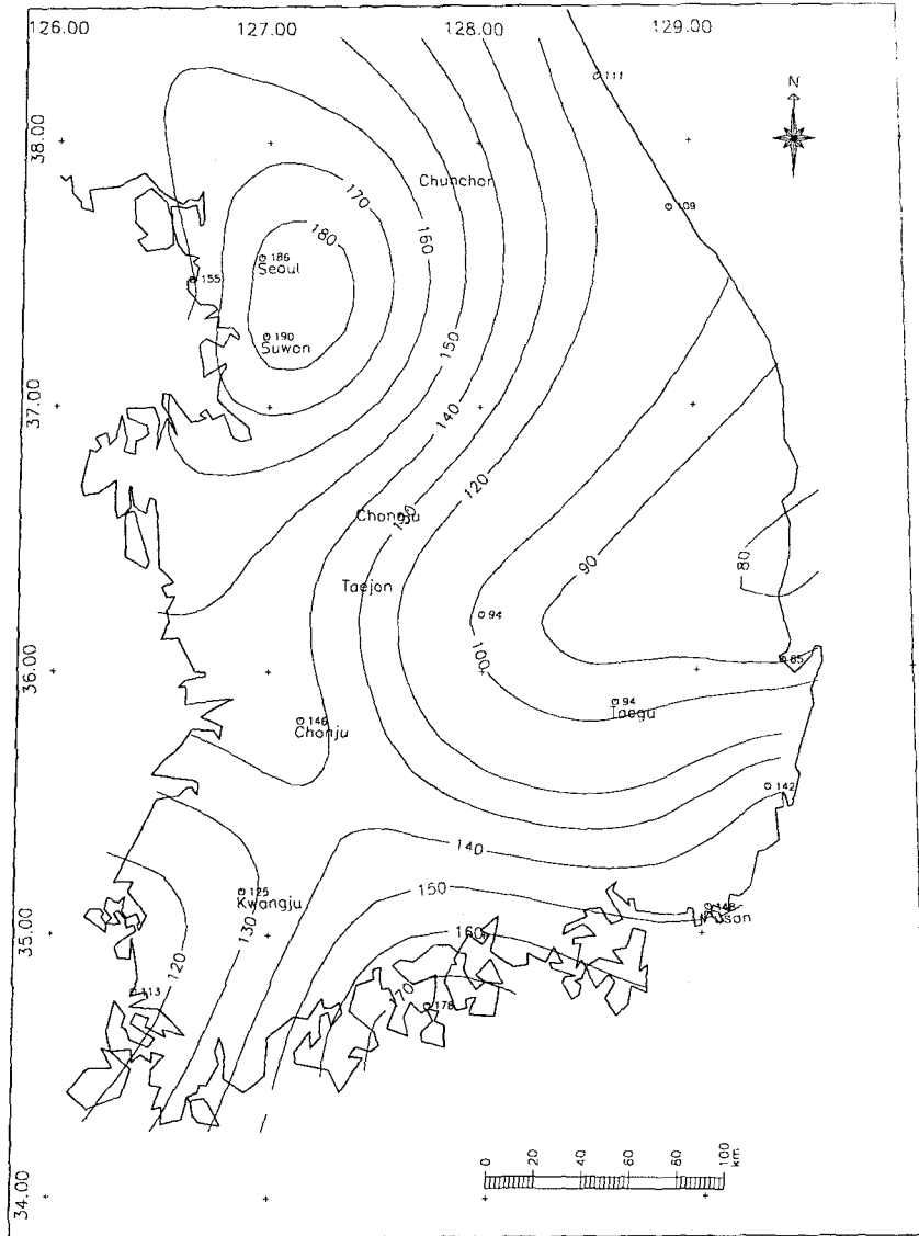
그림 3. 재현기간 2-yr, 지속기간 24-hr 설계호우의 등 R 선도
