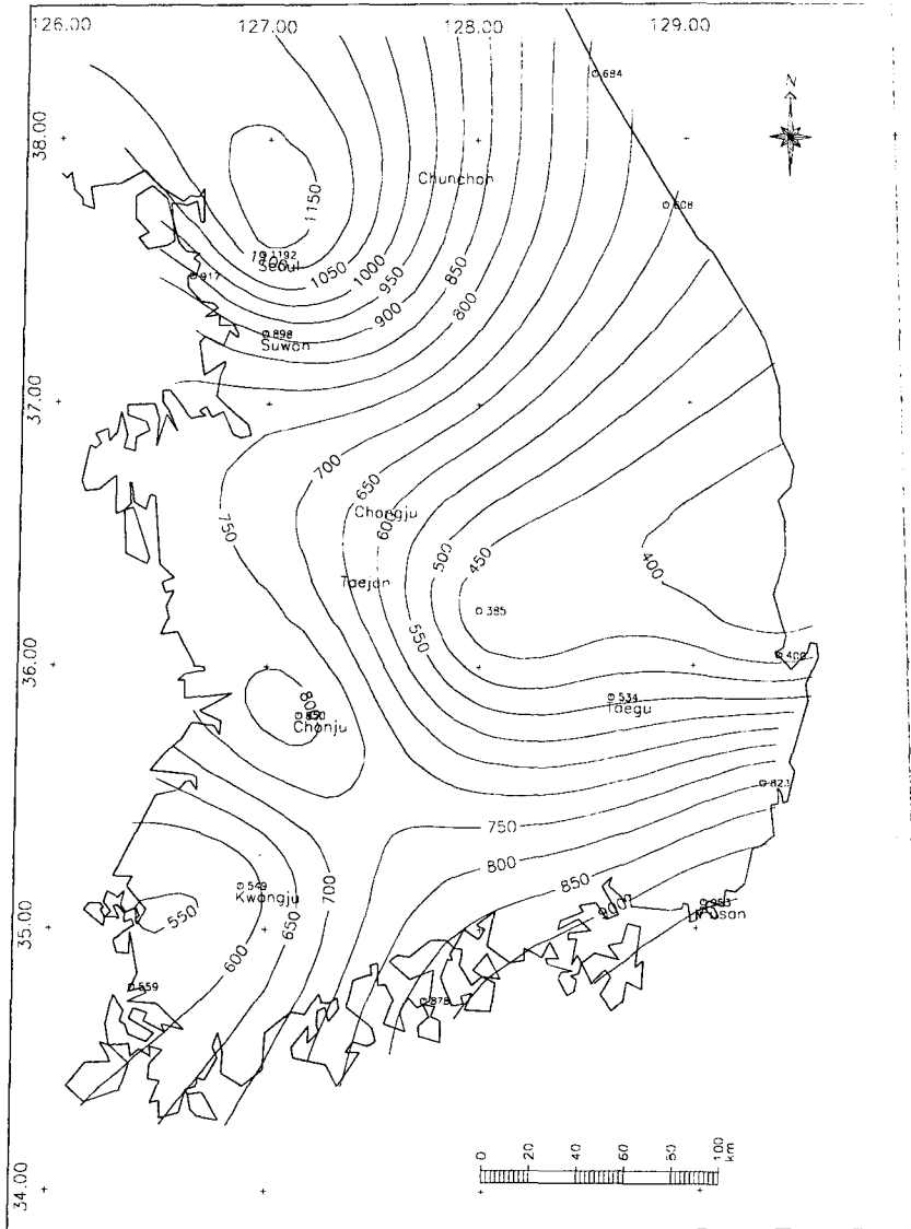
그림 8. 재현기간 50-yr, 지속기간 24-hr 설계호우의 등 R 선도
