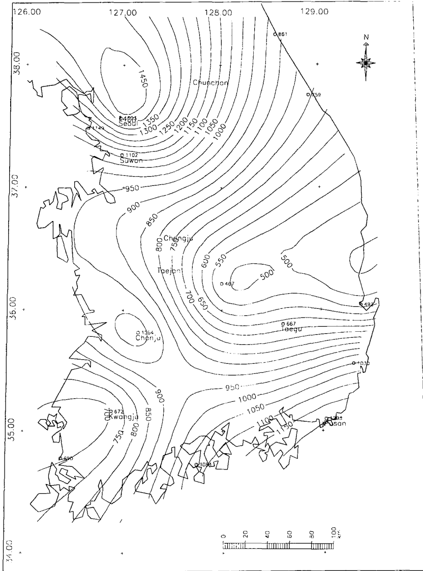
그림 10. 재현기간 100-yr, 지속기간 24-hr 설계호우의 등 R 선도
