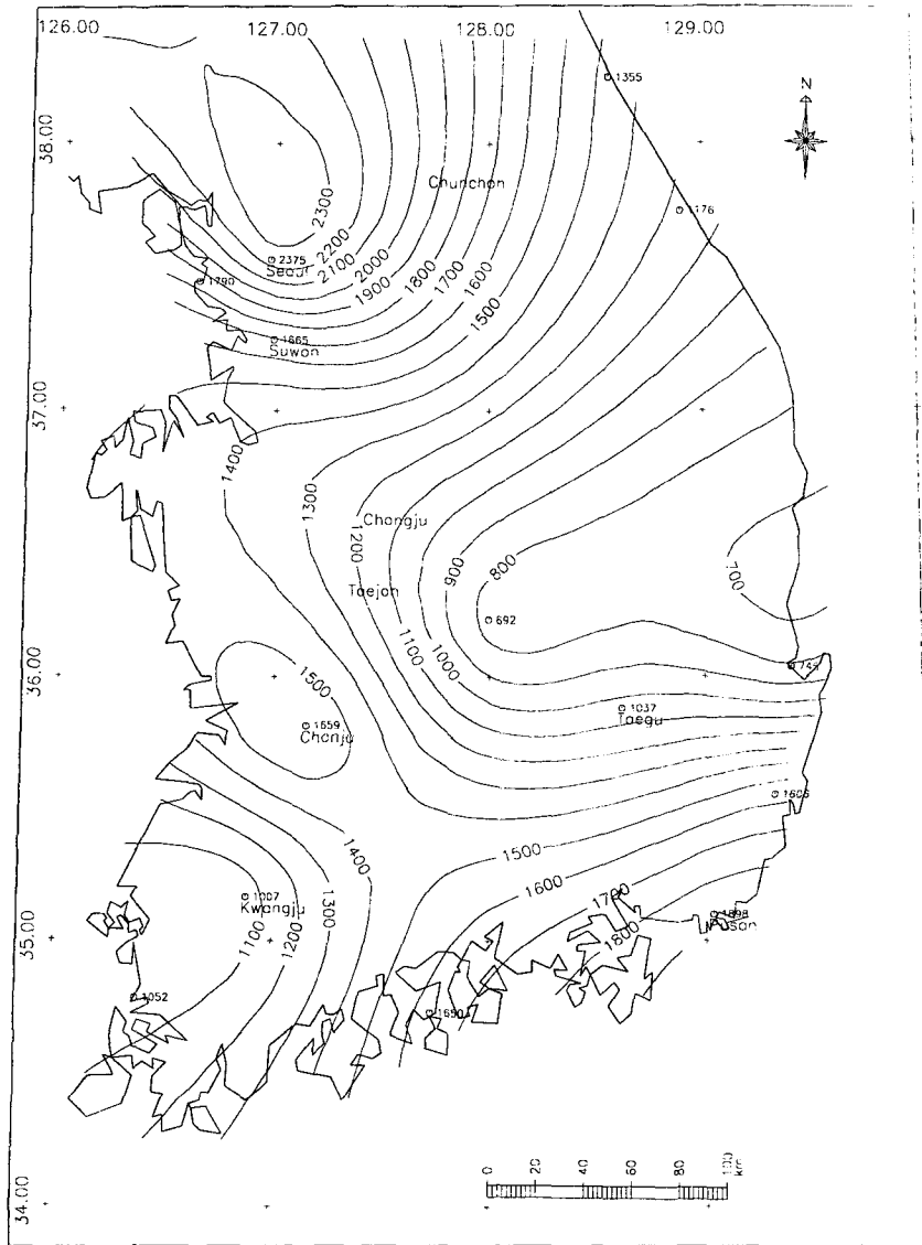
그림 13. 재현기간 500-yr, 지속기간 24-hr 설계호우의 등 R선도
