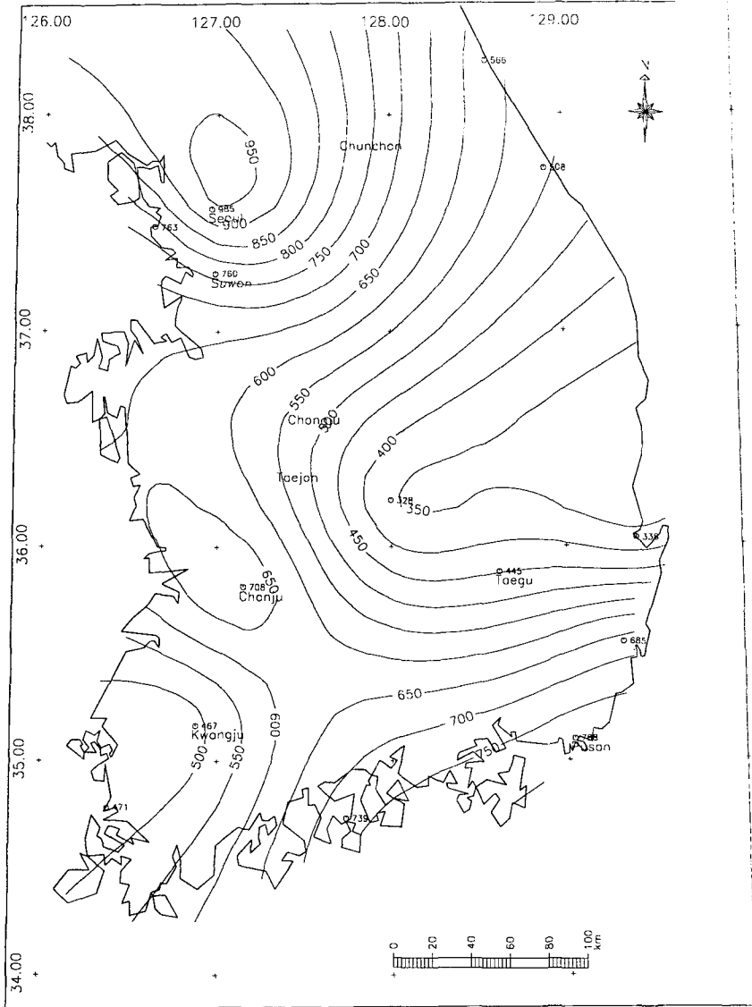
그림 7. 재현기간 30-yr, 지속기간 24-hr 설계호우의 등 R 선도
