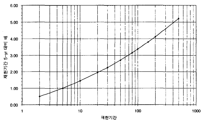
그림 14. 재현기간 5-yr의 R 값 대비 재현기간별 배율
