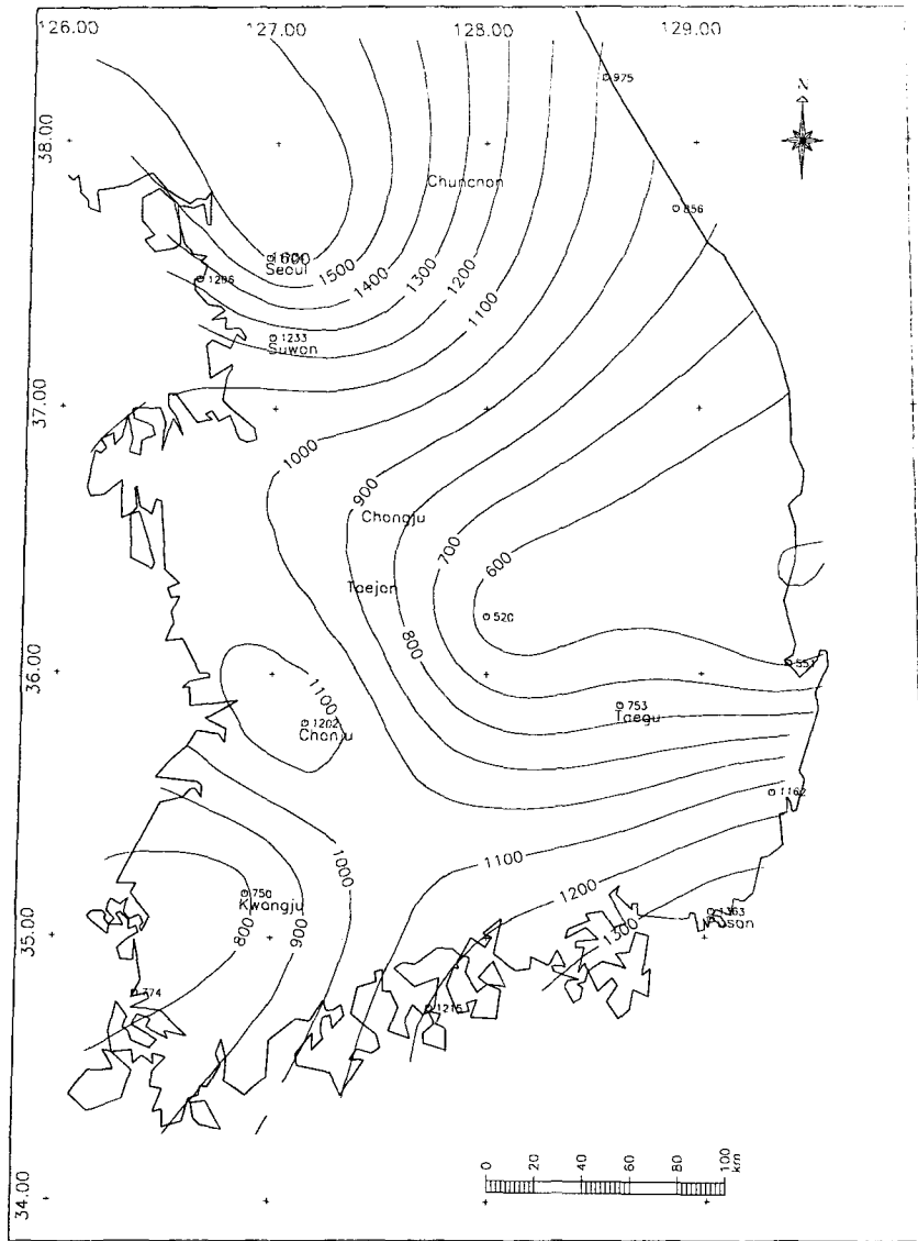
그림 11. 재현기간 150-yr, 지속기간 24-hr 설계호우의 등 R선도
