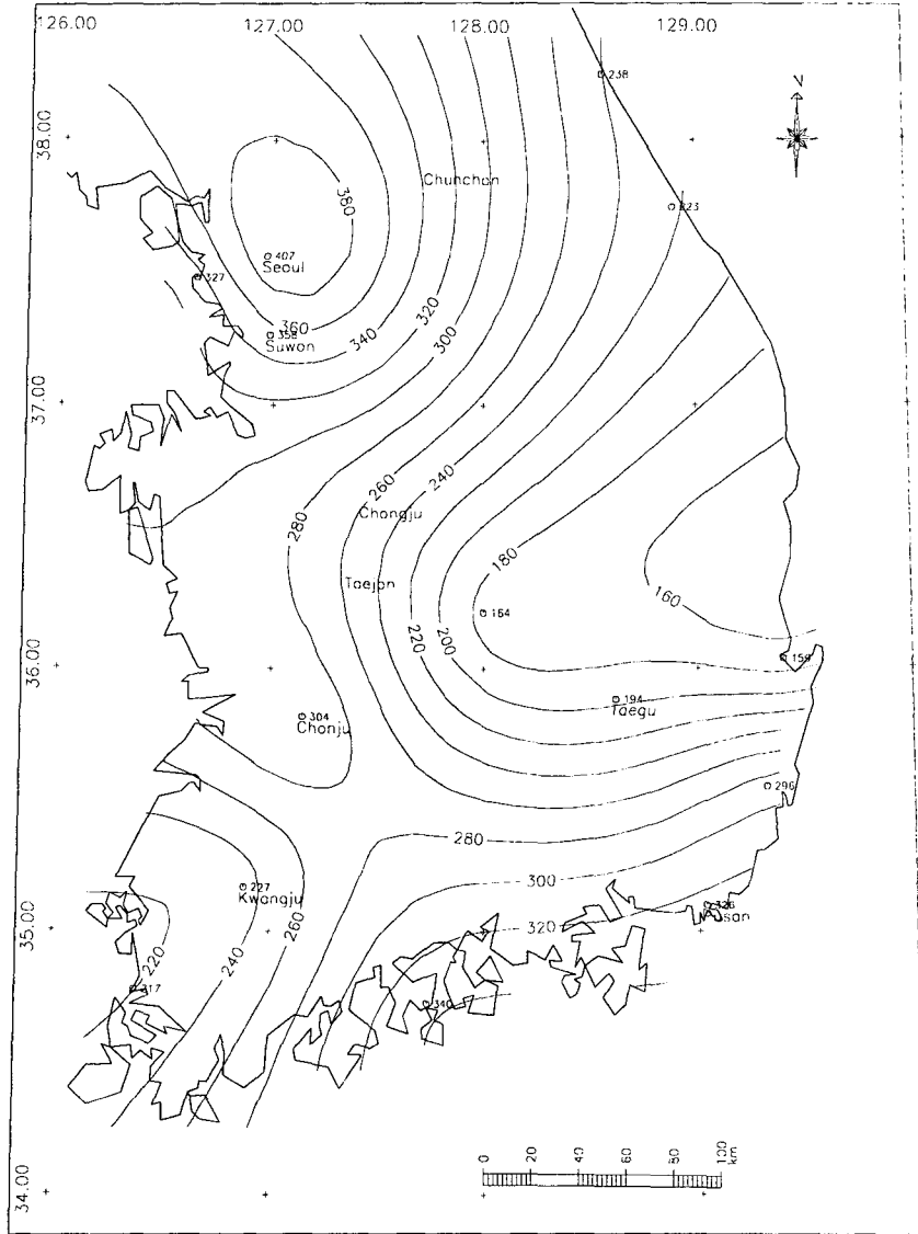
그림 4. 재현기간 5-yr, 지속기간 24-hr 설계호우의 등 R 선도
