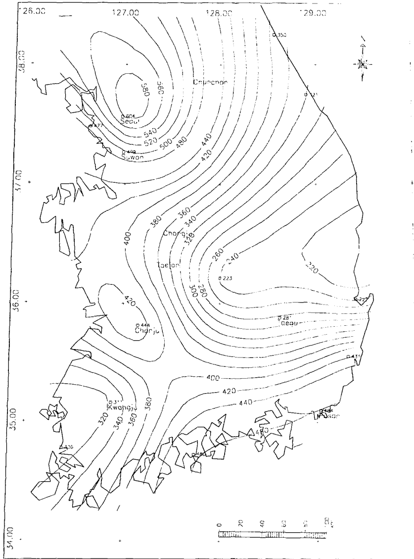
그림 5. 재현기간 10-yr, 지속기간 24-hr 설계호우의 등 R선도
