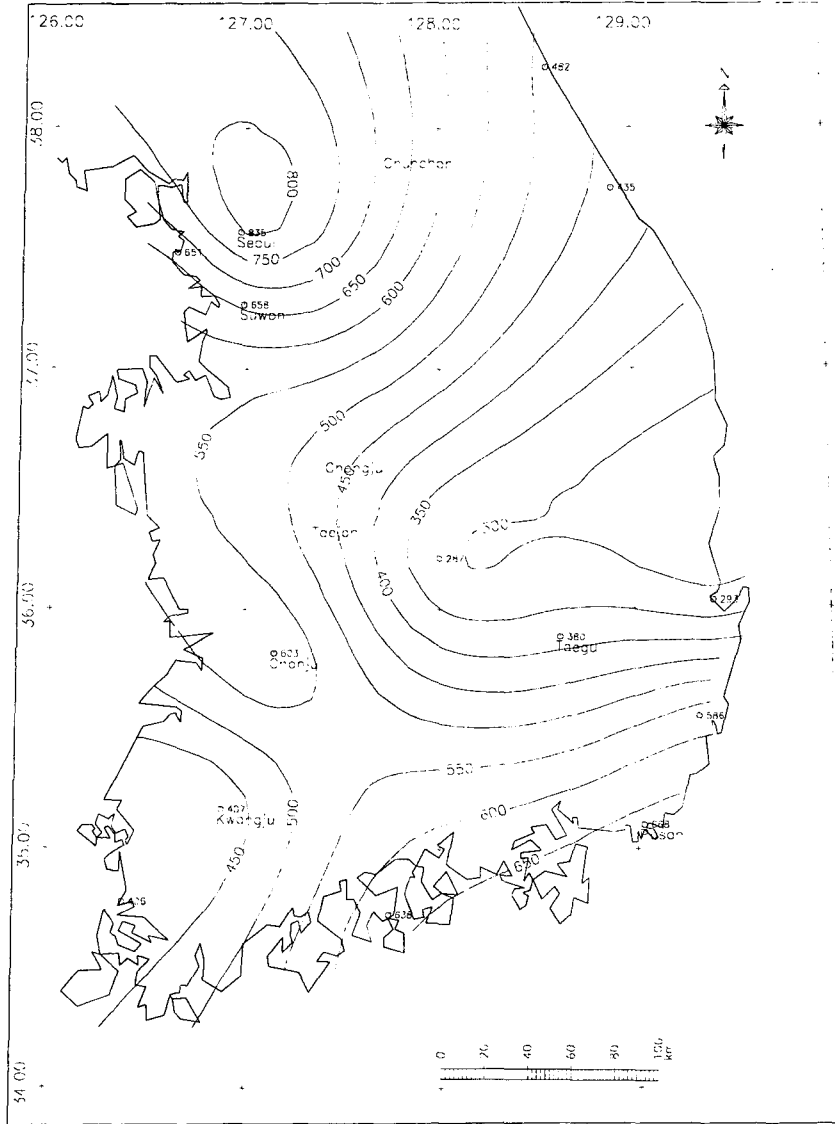
그림 6. 재현기간 20-yr, 지속기간 24-hr 설계호우의 등 R선도
