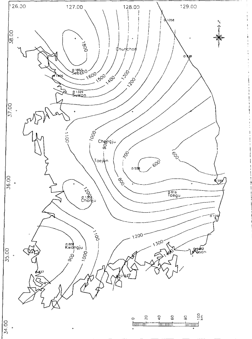
그림 12. 재현기간 200-yr, 지속기간 24-hr 설계호우의 등 R선도
