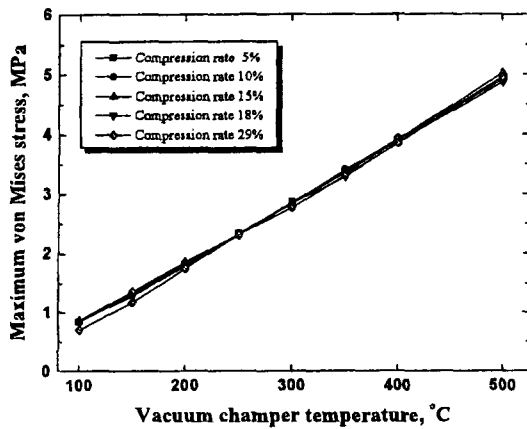
Fig. 8 압축을 변화에 따른 하우징 온도에 의해 발생한 그루브에서의 최대응력
