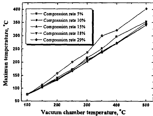
Fig. 3 여러 가지 압축율 변화에 대해 하우스 온도 함수로 제시된 O-링 시일의 최고 온도
