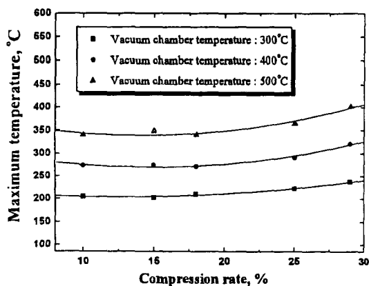
Fig. 4 여러 가지 진공 챔버 온도에 대해 압축율의 함수로 제시된 O-링 시일의 최고 온도
