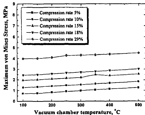
Fig. 6 압축율 변화에 따른 하우징 온도에 의해 발생한 시일에서의 최대응력
