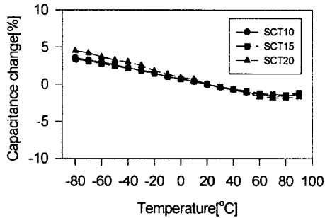
그림 3. 온도에 따른 정전용량의 변화
