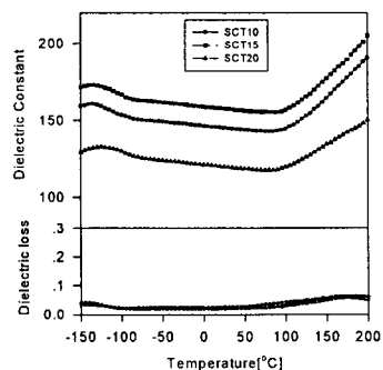
그림 2. SCT 박막의 유전상수와 유전손실의 온도 의존성
