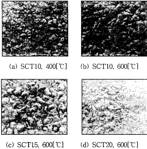
사진 1. SCT 박막의 전자 현미경 사진
