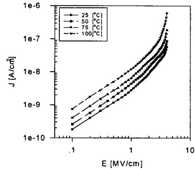
그림 5. 측정온도에 따른 SCT15 박막의 전압-전류 특성
