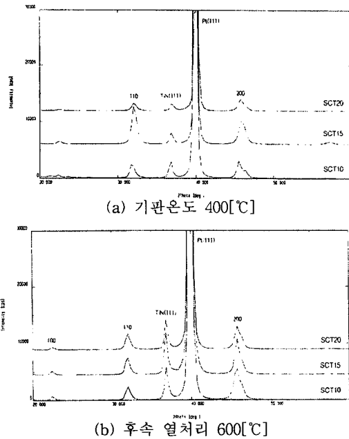
그림 1. SCT 박막의 XRD
