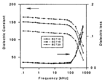
그림 4. 주파수에 따른 SCT 박막의 유전상수 및 유전손실
