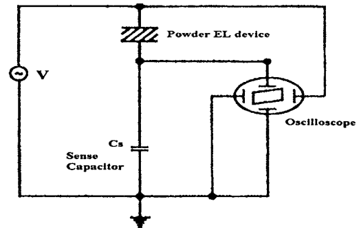
그림 2. Sawyer-Tower's 회로
