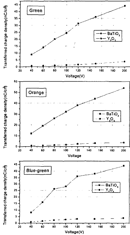
그림7. 전압 변화에 따른 이동전하 밀도
