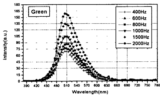
그림3. BaTiO 3 를 사용한 EL소자의 스펙트럼 Figure 3. Spectrum of EL device using the BaTiO 3
