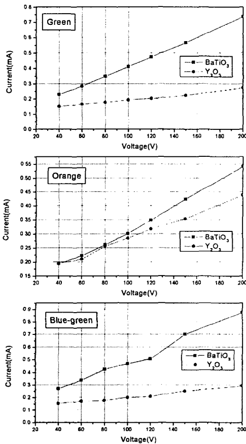
그림6. EL소자의 I-V 특성
