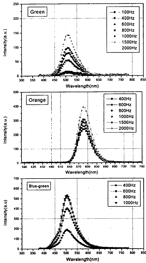
그림3. BaTiO 3 를 사용한 EL소자의 스펙트럼 Figure 3. Spectrum of EL device using the BaTiO 3
