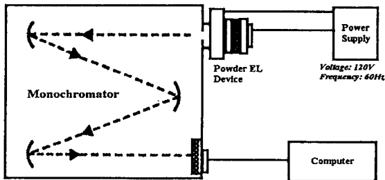
그림 1. EL 스펙트럼 측정 장치도
