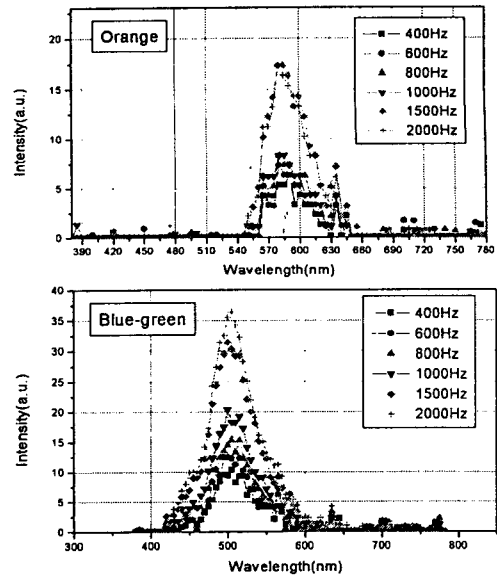
그림4. Y 2 O 3 를 사용한 EL소자의 스펙트럼 Figure 4. Spectrum of EL device using the Y 2 O 3
