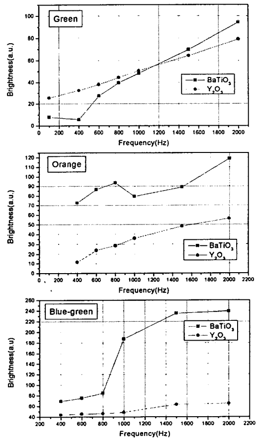
그림5. EL소자의 휘도 특성 Figure 5. Brightness property of EL device
