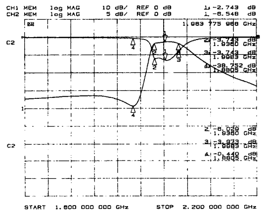
그림 8. 제작된 일체형 유전체 필터의 주파수 전달 특성
