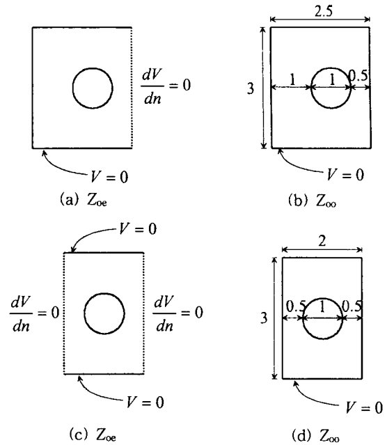
그림 2. Z_{oe} and Z_{oo} 계산을 위한 이차원 FEM 모델 Fig. 2. 2-D FEM models for solving Z_{oe} and Z_{oo}
