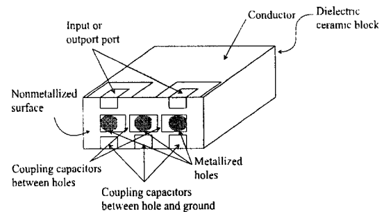
그림 4. 설계된 일체형 유전체 필터의 구조 Fig. 4. Structure for Monoblock dielectric filter
