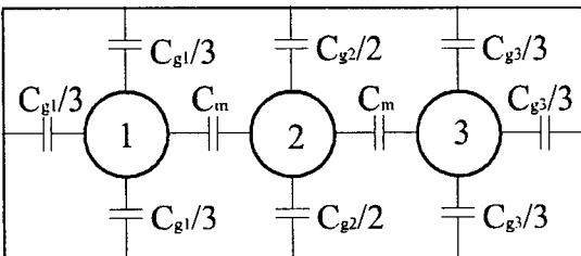
그림 1. 유전체 블록내의 공진홀간의 결합 Fig. 1. Coupled circular cylindrical resonant holes in rectangular ground
