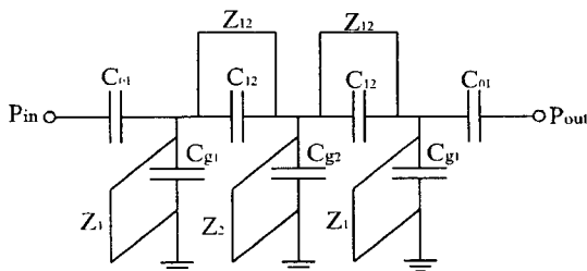
그림 3. 설계된 일체형 유전체 필터의 등가 회로 Fig. 3. Equivalent circuit configuration for the monoblock dielectric BPF
