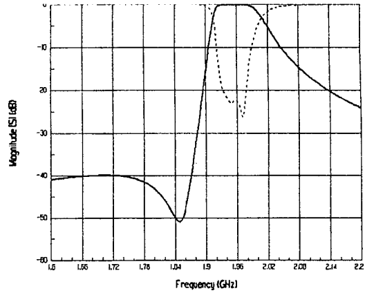
그림 7. 설계된 필터 구조 시뮬레이션 결과 Fig. 7. Structure simulation result
