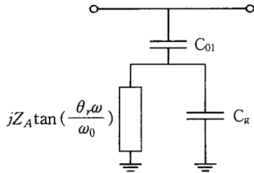
그림 5. C_g 계산을 위한 등가 모델 Fig. 5. Equivalent model for computing C_g
