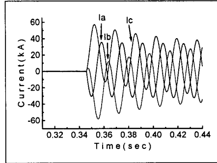
그림 1. 3상 단락사고에 대한 고장전류 파형
