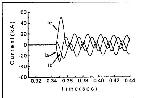
그림 3. 유도형 초전도 한류기를 적용한 3상 단락사고 (사고각 0°)
