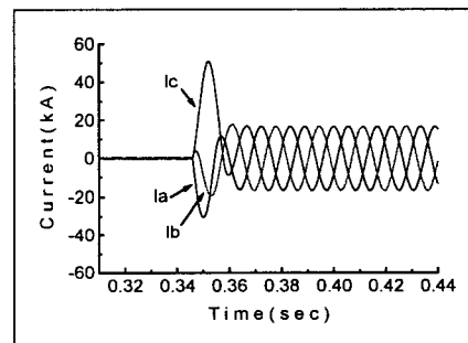
그림 2. 저항형 초전도 한류기를 적용한 3상 단락사고 (사고각 0^\circ )
