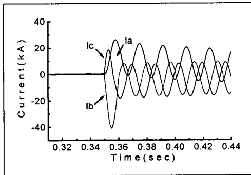
그림 7. 유도형 초전도 한류기를 적용한 3상 단락사고 (사고각 90°)
