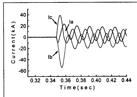
그림 5. 유도형 초전도 한류기를 적용한 3상 단락사고 (사고각 45°)
