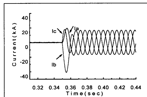
그림 6. 저항형 초전도 한류기를 적용한 3상 단락사고 (사고각 90°)
