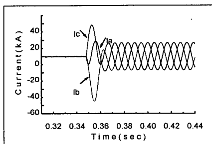
그림 4. 저항형 초전도 한류기를 적용한 3상 단락사고 (사고각 45°)
