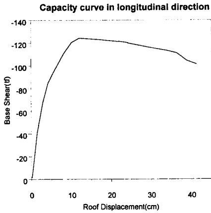
그림 4 역량곡선(Capacity Curve)
