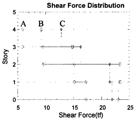
그림 7 중앙기둥의 전단력 도
