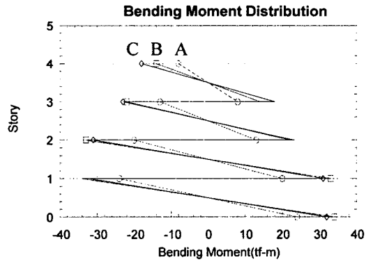
그림 8 중앙기둥의 모멘트 도
