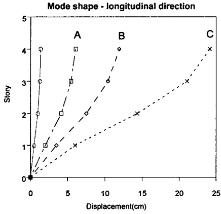
그림 6 중앙기둥의 변형형상
