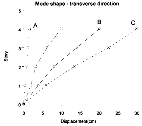
그림 6 중앙기둥의 변형형상
