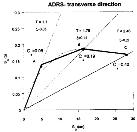
그림 5 ADRS 스펙트럼
