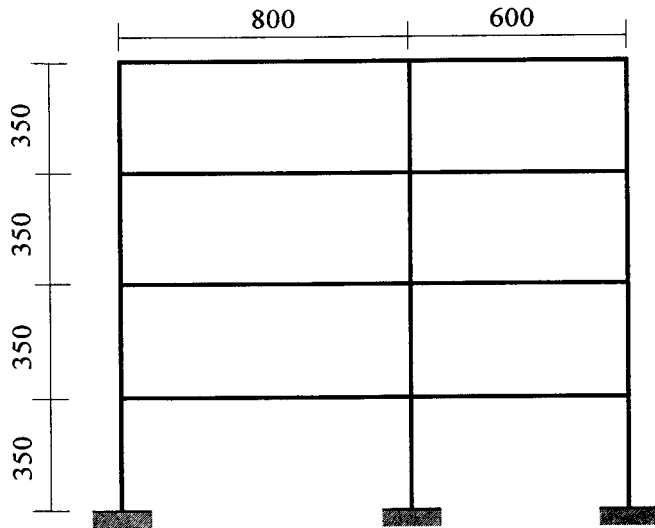
그림 2 모델 건축물의 입면도
