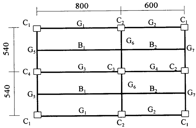
그림 1 모델 건축물의 평면도
