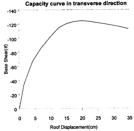
그림 4 역량곡선(Capacity Curve)
