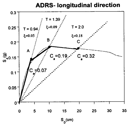
그림 5 ADRS 스펙트럼
