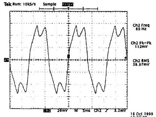
그림 3. 입력 전류 파형 Fig 3. Input current wave form
