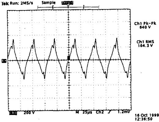
그림 5. 저압나트륨 램프의 관 전압 Fig 5. Lamp voltage of low pressure sodium lamp
