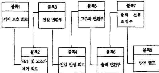
그림 1. 저압 나트륨 램프용 고효율 전자식 안정기 블록도
