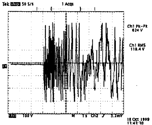
그림 4. 전자식 안정기의 시동 전압 Fig 4. Starting voltage of electronic ballast
