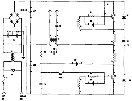
그림 2. 저압 나트륨 램프용 고효율 전자식 안정기 회로도
