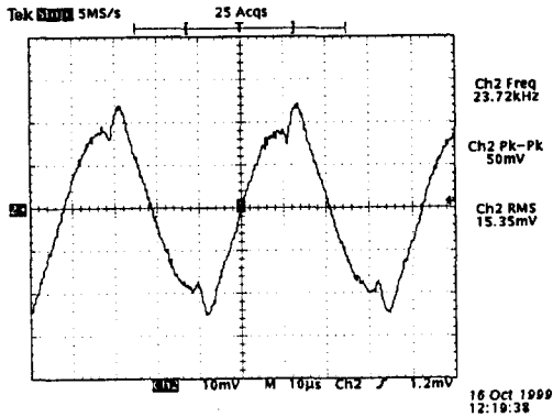
그림 6. 저압 나트륨 램프의 관 전류 Fig 6. Lamp current of low pressure sodium lamp
