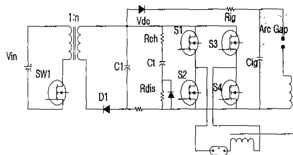
그림 1. 기존의 HID 안정기 시스템
