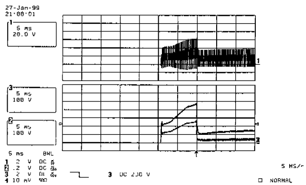
b) 제안된 시스템 (최대 Vdc:280V, 최대 Vdsp:60V)
