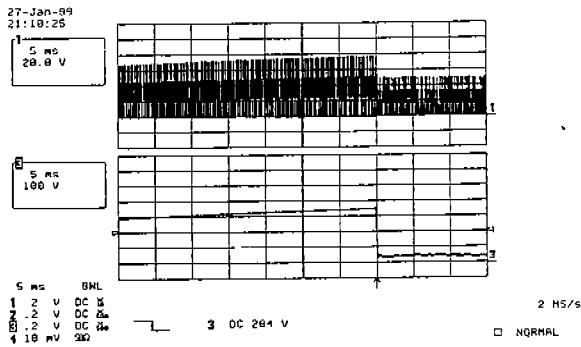
a) 기존 안정기 (Max Vdc:350V, Max Vdsp:80V)
