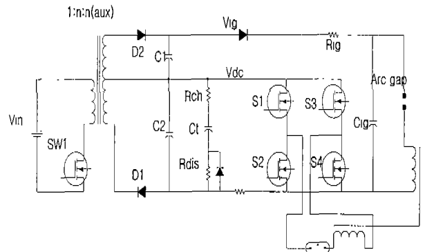
그림 2. 제안된 HID 안정기 시스템
