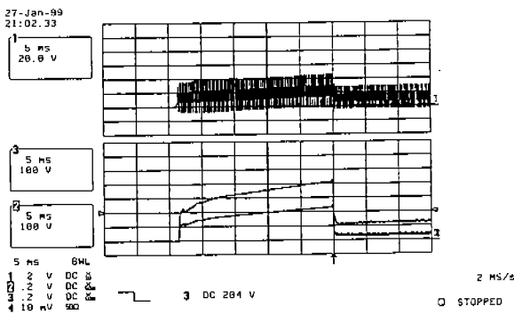
b) 제한된 시스템 (Max Vdc:250V, Max Vdsp:50V)
