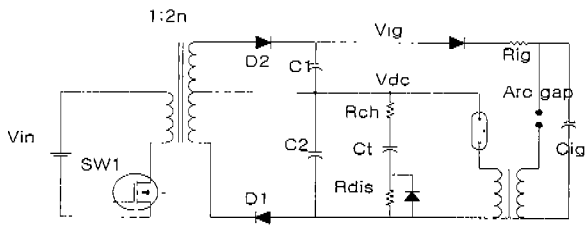
a) 점등전 상태
