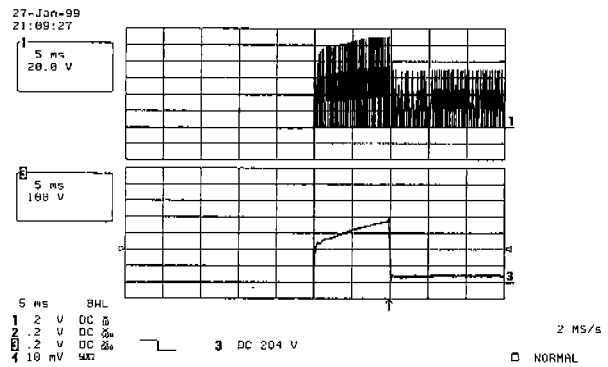
a) 기존 안정기 (최대 Vdc:400V, 최대 Vdsp:90V)
