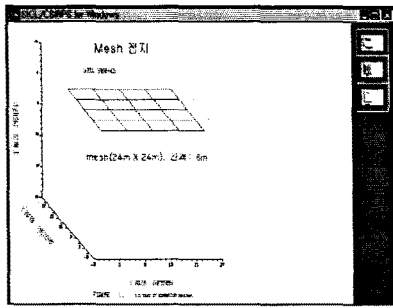
그림. 2-5 매쉬접지 설계 구조
