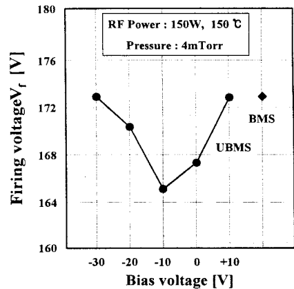
그림 6. 기판 Bias 전압에 따른 방전개시전압
