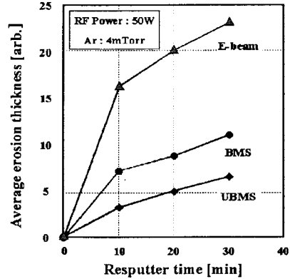
그림 9. MgO 제작 방법에 따른 내스퍼터링 특성
