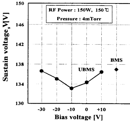
그림 7. 기판 Bias 전압에 따른 방전유지전압
