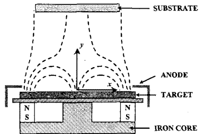
그림 2. 불평형 마그네트론 스파터링의 개략도
