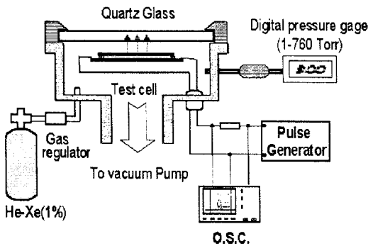
그림 4. 방전 챔버의 개략도
