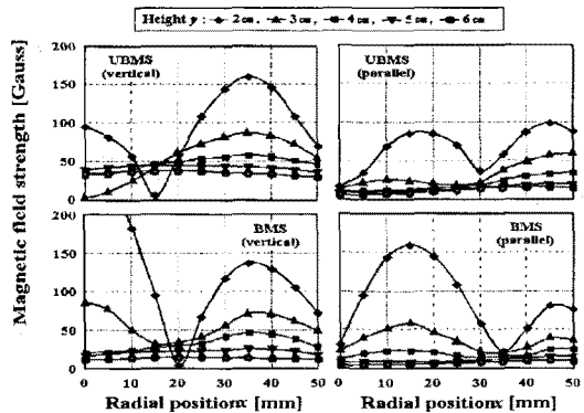
그림 3. UBMS와 BMS의 수직, 수평 자력선 강도
