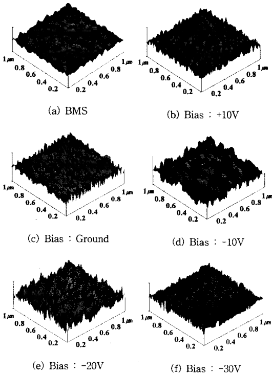
그림 8. 기판 bias 전압에 따른 MgO 표면 AFM 사진
