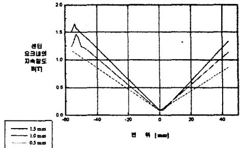
그림 4. 중심요크내의 자속밀도분포( t_c=6.0mm )
