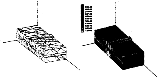
(a) LDM의 요소망 및 자속밀도 분포도
