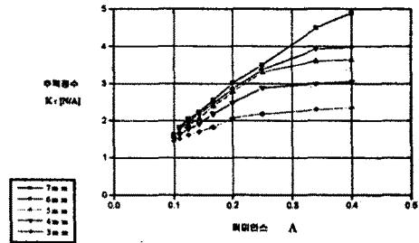
그림 3. 자계해석(FEM)에 의한 추력정수( t_c=1.0mm )
