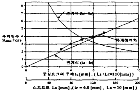
그림5. 추력정수와 중심요크 두께 및 스트로크의 관계
