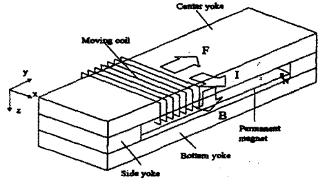
그림 1. 가동코일형 LDM의 구조 및 추력발생원리
