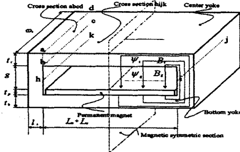
그림 2. 가동코일형 LDM의 자속흐름 개념도
