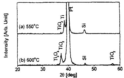
그림 2 열처리 온도에 따른 Pt/Ti/SiO 2 /Si 기관의 변화
