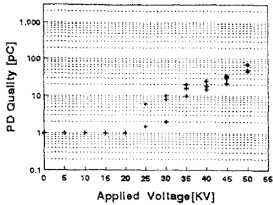
그림 2. A3 제품의 PD 측정.
