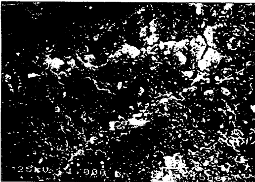
사진 1. EPDM 애자의 트래킹열화
