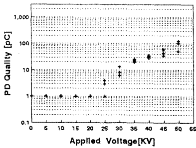
그림 3. B1 제품의 PD 측정.
