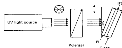
그림 2. 실험에 사용한 UV 광의 조사장치.
