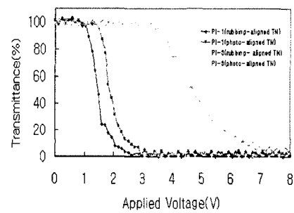
그림 4 CF 3 기를 함유한 가용성 폴리이미드 표면에 직선 편광된 UV광을 20°의 입사각도로 20분간 조사한 광배향 TN-LCD와 러빙처리한 TN-LCD와의 V-T 특성.
