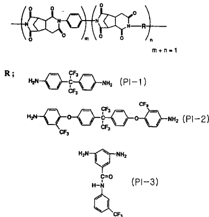
그림 1. 사용한 3 종류의 폴리머의 분자구조.
