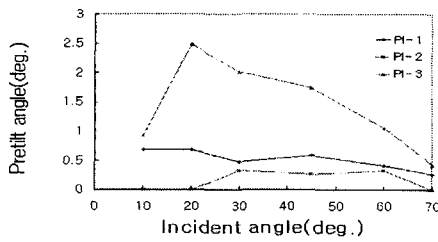
그림 3. CF 3 기를 함유한 3 종류의 가용성 폴리이미드 표면에 직선 편광된 UV 광을 20분간 경사 조사시의 프리틸트각의 입사각도 의존성.
