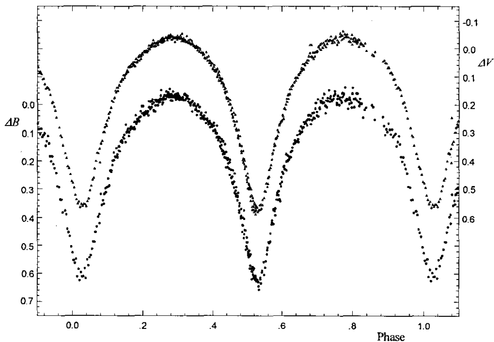
Figure 1. BV light curves of ER Orionis.
