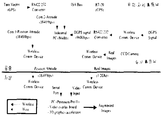
그림 3 단위시스템의 연결도
