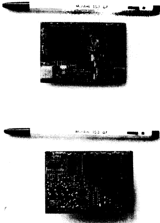
그림 2. \mu -law PCM 코덱을 사용하고 훈련데이터 보존을 위한 배터리 Backup 기능을 가진 VR32 음성인식 모듈의 앞면과 뒷면 사진
