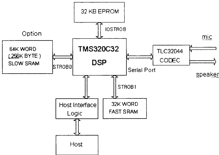
그림 1. VR32의 하드웨어 구성도
