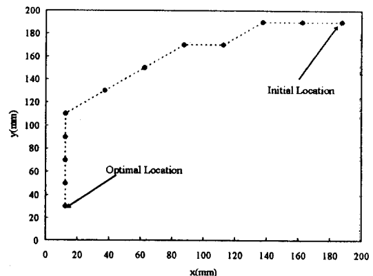
Fig. 4 Optimization using Gradient Method for [45_4/0_2/90_2] Plate(S/A length=25 mm)
