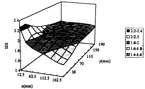
Fig. 3 SDI of [45_4/0_2/90_2] Plate(S/A length=25 mm)
