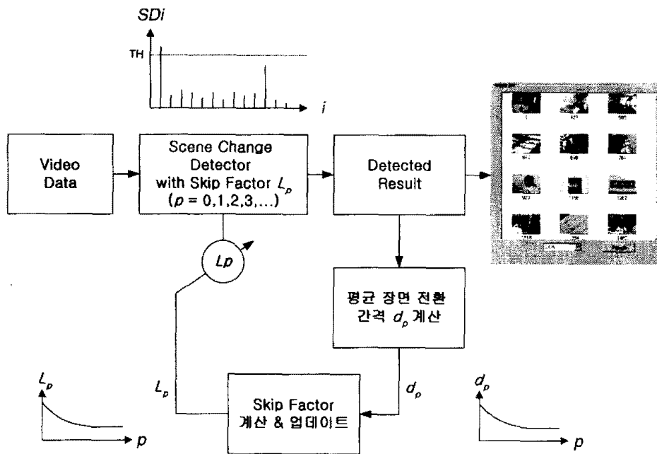
그림 9: 최적 검출 간격 장면 전환 검출
