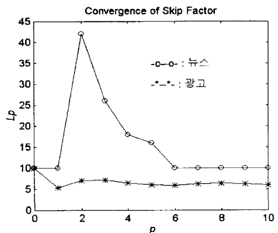
그림 11: 검출 간격의 수렴 형태
