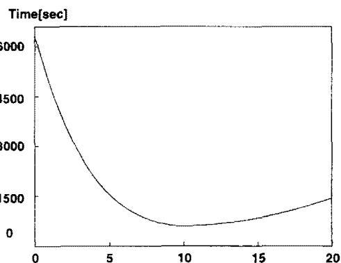
그림 4: 검출 간격과 검출 시간의 관계
