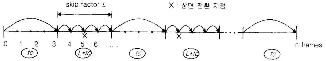
그림 5: 검색 간격 L 로 장면 전환 검출하는 형태
