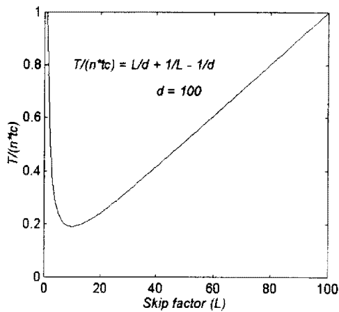
그림 6: T/(n \times t_c) = L/d + 1/L - 1/d
