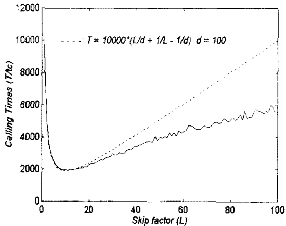
그림 8: 이상적인 동영상의 경우 검색 시간
