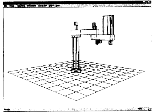
그림 10. 와이어 프레임 모델
