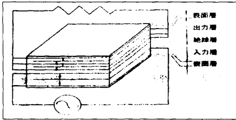
<그림 6> 두께중진동형 압전트랜스 구조
