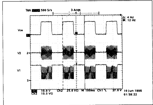
<그림 4> 저주파수에서의 스위칭 파형.
