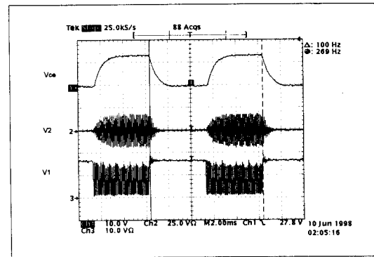
<그림 5> 스위칭이 원활하지 못한 파형
