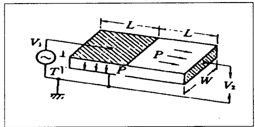
<그림 1> 3단자 구조의 Rosen형 압전트랜스
