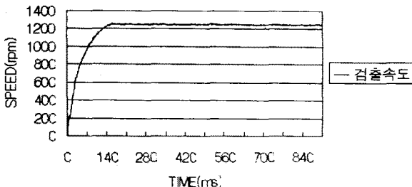
그림 5 피지제어를 사용한 계단응답
