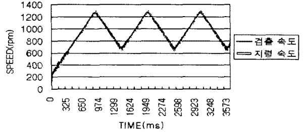
그림 7 삼각파 속도지령을 주었을 때의 속도응답
