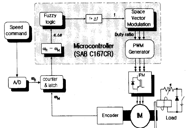
그림 1 시스템의 전체 구성도
