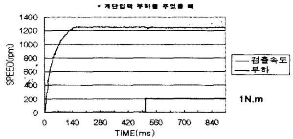
그림 6 부하를 주었을 때의 계단응답
