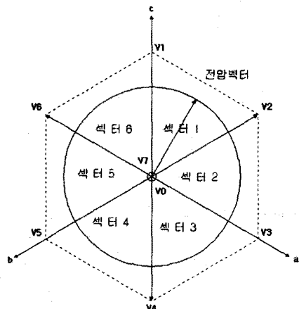
그림 4 평면상의 전압벡터의 제적
