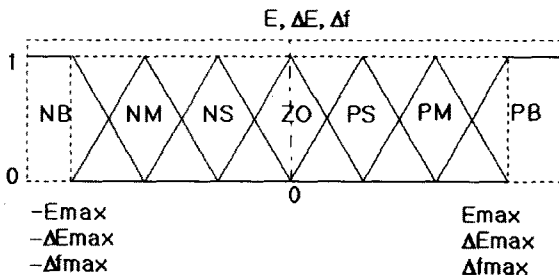
그림 2 멤버쉽 함수
