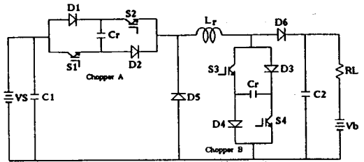
그림3. 소프트 스위칭에 의한 승압 초퍼회로
