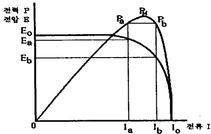
그림. 1 태양전지 출력특성
