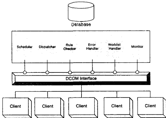
<그림 8> 시스템구조
