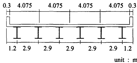
그림 1 대상교량의 단면
