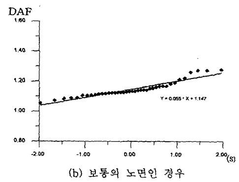
그림 4 43.2ton 세미트레일러에 의한 응답확대계수의 확률분포특성
