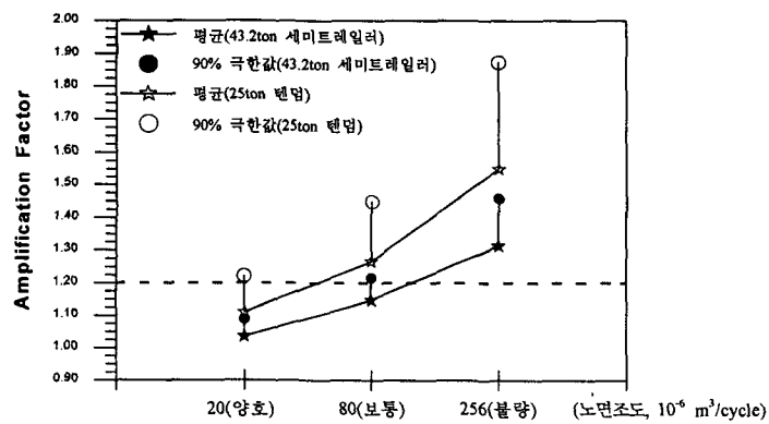
그림 5 노면조도에 따른 응답확대계수
