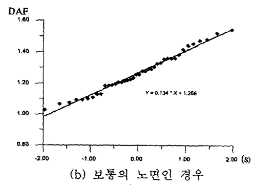
그림 3 25ton 텐덤축트럭에 의한 응답확대계수의 확률분포특성
