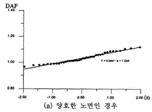
그림 3 25ton 텐덤축트럭에 의한 응답확대계수의 확률분포특성
