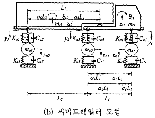
그림 2 차량모형
