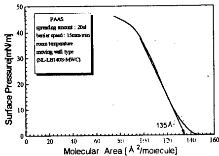
그림 4. PAAS의 \pi -A isotherm.
