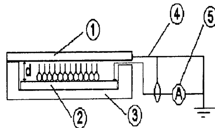
① 상부 전극 ② 하부 전극 ③ BN block ④ 금 선 ⑤ 전류계
