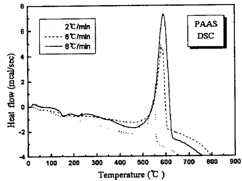
그림 6. PAAS의 DSC 측정.
