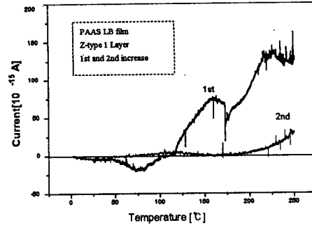
(b) 열자극 전류 측정
