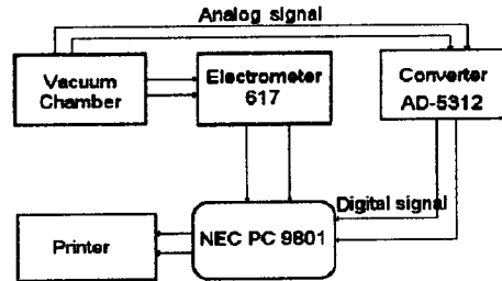
그림 2. 열자격 전류 측정 장비의 블록 선도.
