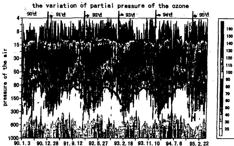
그림1. 쓰꾸바 상공에서의 오존의 시간 및 고도에 따른 분포도. 수치는 오존의 부분압( 10^{-6} hpa)이고, y축은 대기의압력(고도에 해당), 그림 중앙에 있는 굵은선은 본인이 입수 가능했던 시기의 대류 권계면의 고도를 나타낸다.
