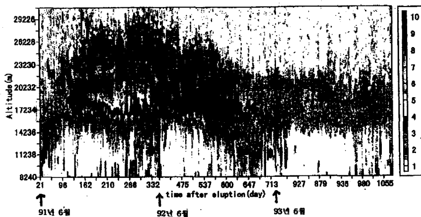
그림3. 필리핀의 피나투보 화산의 분화 후, 도쿄카와의 라이다로 관측한 고층의 에어로졸의 분포도. x축은 91년 6월의 분화일로부터의 경과 일수이다.
