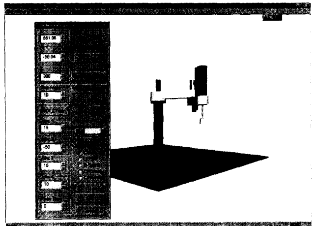
그림 5. 교시 대화 상자에서의 경유점 정보 입력 Fig.5. Input Via_Point information in Teach Dialog Box
