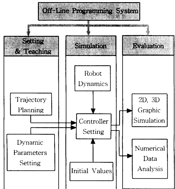
그림 1. OLP 시스템의 구성
