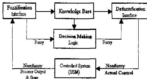
그림 5. 퍼지논리제어기의 기본 구성도
