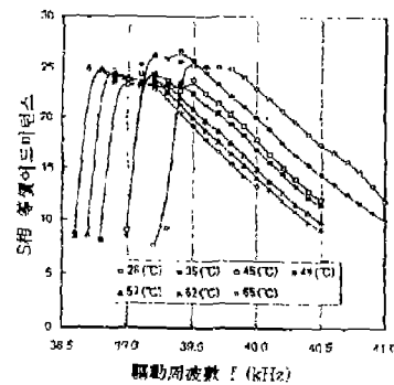
그림 4. USM의 온도에 따른 주파수 특성
