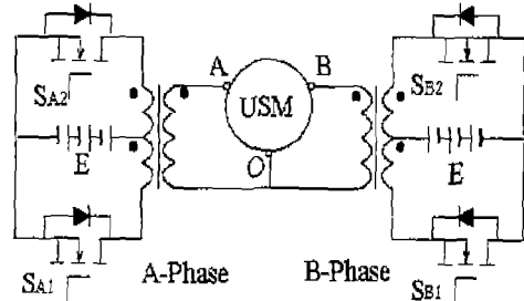
그림 3. 초음파 모터 구동용 공진형 인버터
