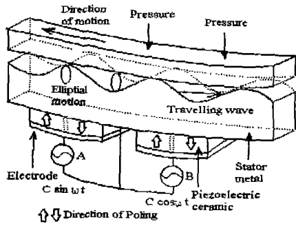
그림 2. 진행파형 모터의 원리
