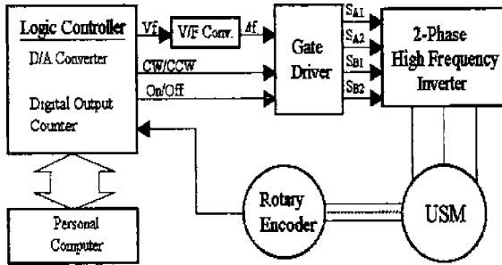
그림 7. 제어시스템
