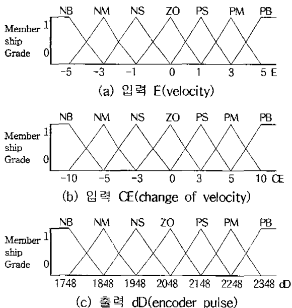
그림 6. 초음파 모터의 소속함수
