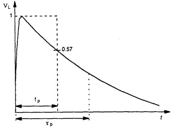
그림 2. 장치의 이론적 특성 곡형
