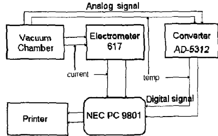
그림 2. 열자극 전류 측정 장비의 블록 선도.
