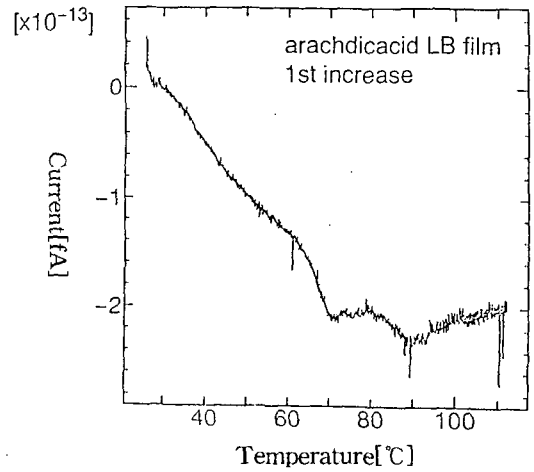
그림 6. Arachidic acid(AA) LB 박막의 열자극 전류 측정.
