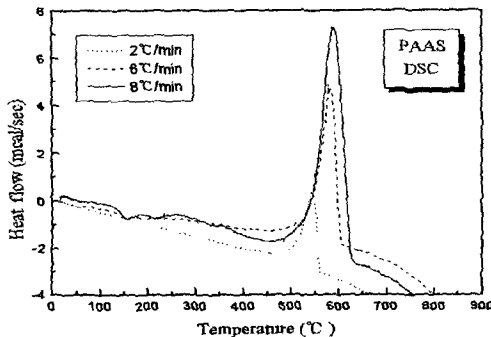
그림 9. PAAS의 DSC 측정.
