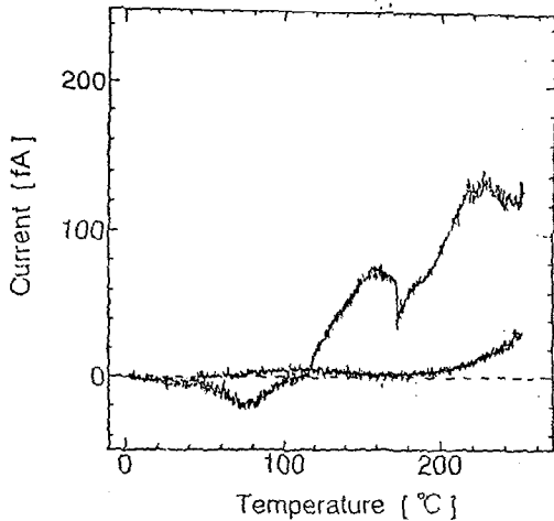
그림 8. PAAS LB 박막의 열자극 전류 측정.
