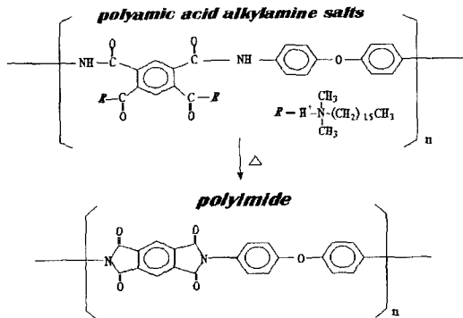
그림 1. 성막 분자의 구조.
