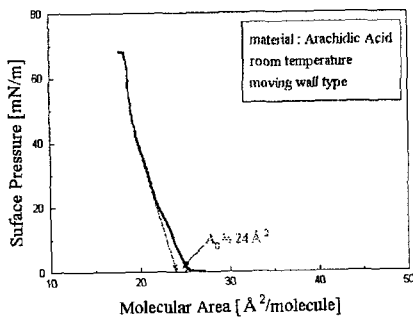
그림 4. Arachidic acid(AA)의 \pi -A isotherm.
