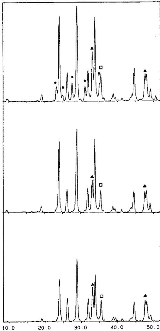
그림 4 가공-열처리 공정에 따른 XRD 분석 ● Bi2212, □ CuO, ▲ Bi2212+Bi2223
