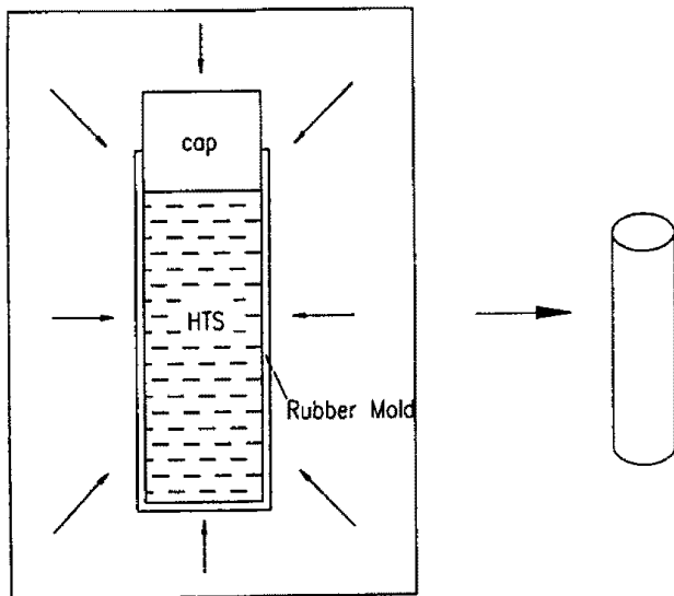
그림 1 정수압프레스에 의한 전류도입선 성형
