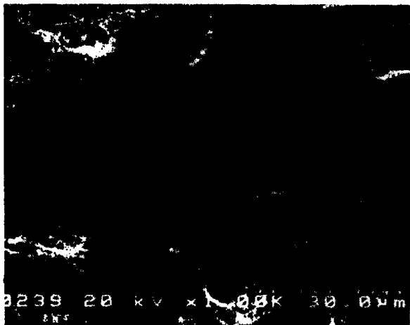
그림 7 CIP 성형과 저산소 분위기, 836°C에서 80 시간 열처리를 3번 반복한 Bi2223 시료에서의 SEM 조사
