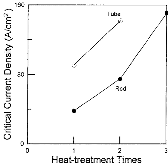
그림 3 가공-열처리 공정에 따른 전류밀도 변화
