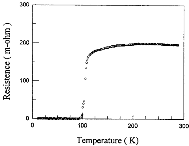
그림 6 저산소 분위기, 842°C에서 80 시간 열처리한 Bi2223 시료의 임계온도 Tc 조사
