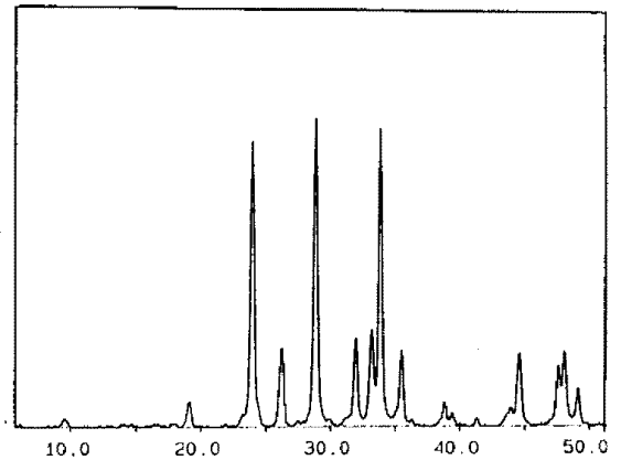
그림 5 저산소 분위기, 842 °C에서 80 시간 열처리한 Bi2223 시료의 XRD 조사
