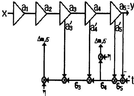
< 그림 2 > FNN의 블록 다이어그램
