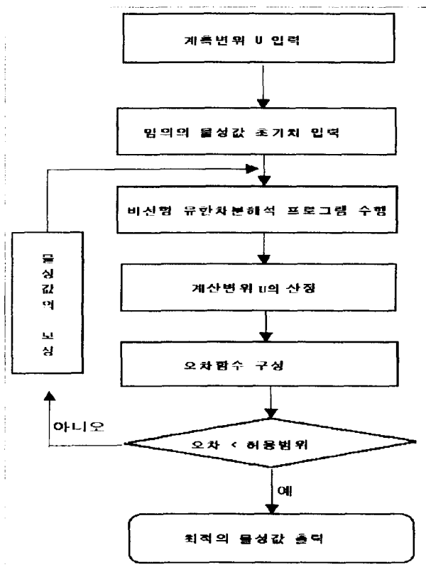
그림 1. 역해석 과정의 흐름도
