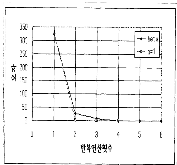
그림 11. 오차의 수렴과정
