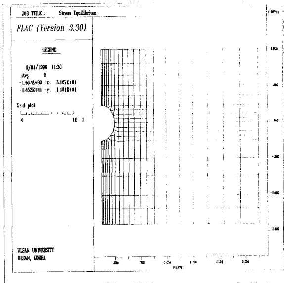
그림 2. 정해석의 모델링
