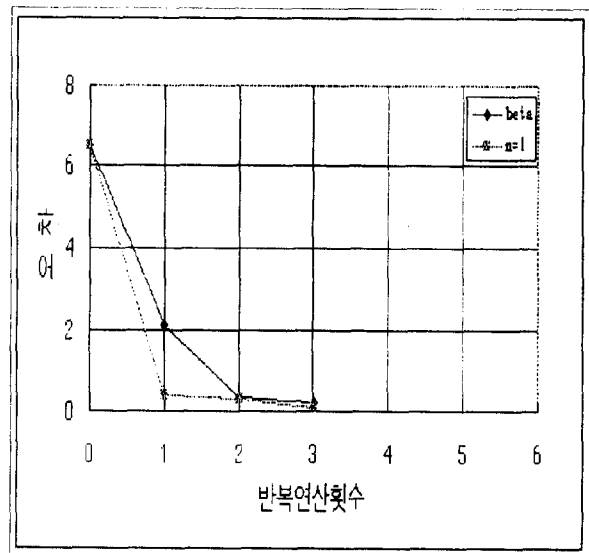
그림 13. 오차의 수렴과정
