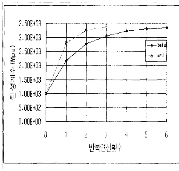
그림 10. 탄성계수의 역해석 결과(계측점수가 1개)
