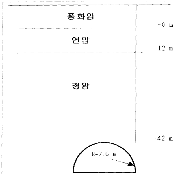
그림 8. 역해석 대상의 횡단면도
