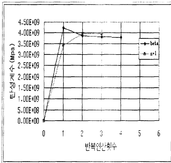
그림 12. 탄성계수의 역해석 결과(계측점수 2개)
