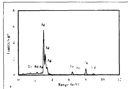
Fig. 10. 웅착마모입자의 형상과 성분
