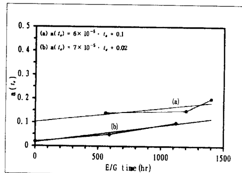
Fig. 5. 엔진 사용시간에 대한 기울기의 변화
