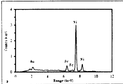
Fig. 11. 절삭마모입자의 형상과 성분
