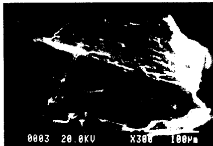
Fig. 11. 절삭마모입자의 형상과 성분
