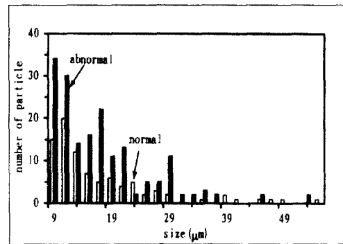
Fig. 6. 정상 및 비정상 상태 엔진의 오일내 마모입자 분포( >8\mu\text{m} )
