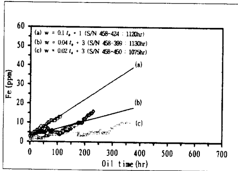
Fig. 3. 오일 사용시간에 대한 Fe 마모입자 농도(엔진 사용시간 : 1000hr이상)
