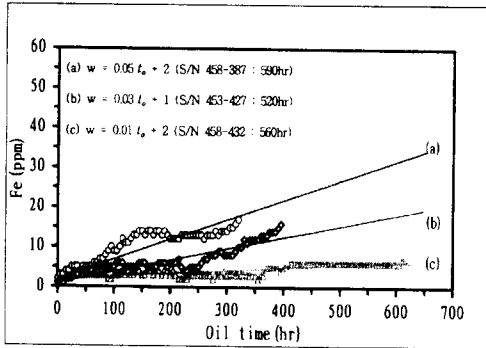
Fig. 2. 오일 사용시간에 대한 Fe 마모입자 농도(엔진 사용시간 : 500-1000 hr)
