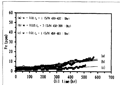
Fig. 1. 오일 사용시간에 대한 Fe 마모입자 농도(엔진 사용시간 : 500hr이하)
