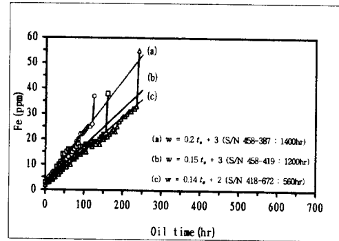
Fig. 4. 오일 사용시간에 대한 Fe 마모입자 농도
