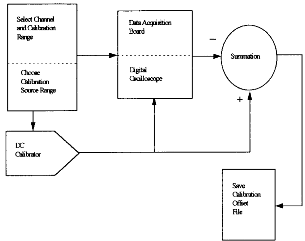
그림 8. 장비오차보정 알고리즘
