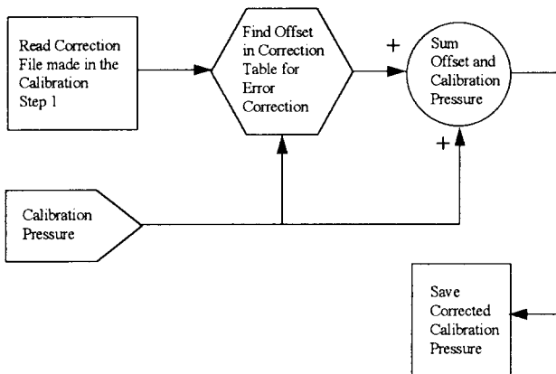
그림 7. 압력오차보정 알고리즘
