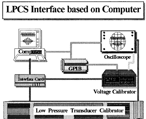
그림 9. 교정시스템 블록다이어그램
