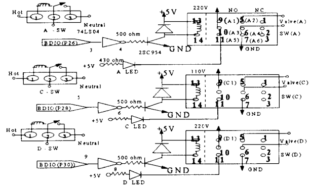
그림 4. 제어용 인터페이스 회로 Fig. 4. Interface circuit for control
