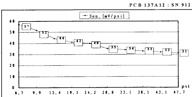
그림 11. 교정 감도표
