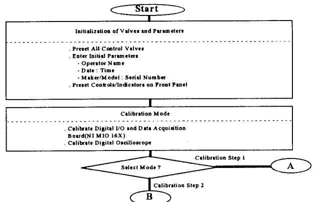
그림 5. 교정시스템 동작 과정 Fig. 5. Operation process of CAL. system
