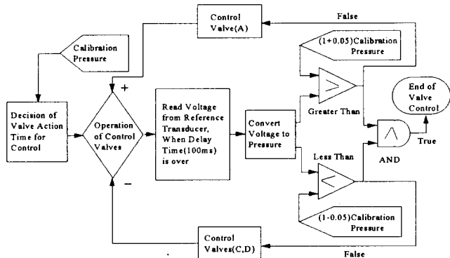
그림 6. 자동압력제어의 블록다이어그램
