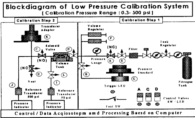
그림 2. 교정기 블록다이어그램 Fig. 2. Block diagram of the calibrator
