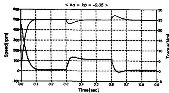
(a) 속도와 토크
