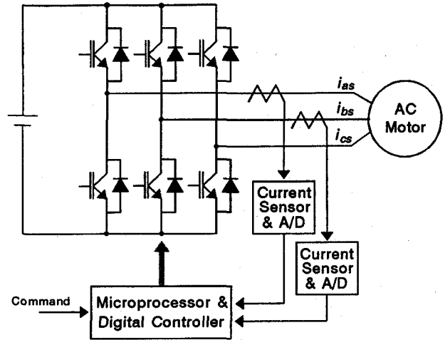
그림 1. 인버터에 의한 교류전동기 구동시스템
