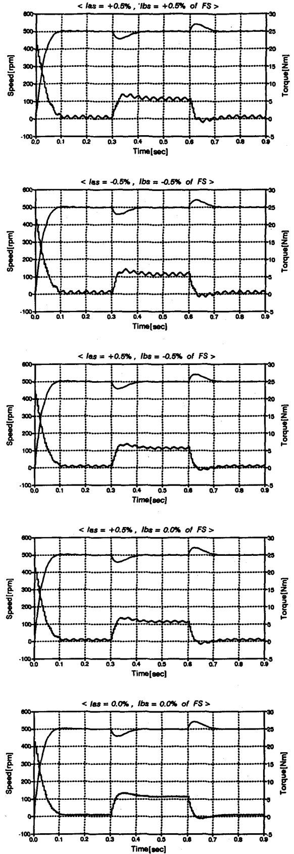
그림 2. 오프셋 전압에 기인하는 토크리플 및 이를 제거한 경우의 시뮬레이션 결과
