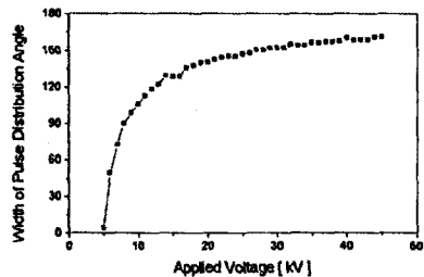
그림 3.5 PD펄스의 위상각 분포
