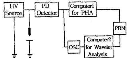
그림 2.1 부분 방전 측정 및 Wavelet 해석 시스템
