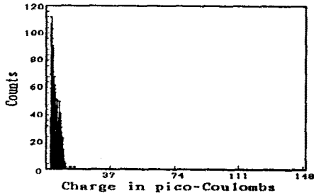
그림 3.1 PD펄스의 히스토그램
