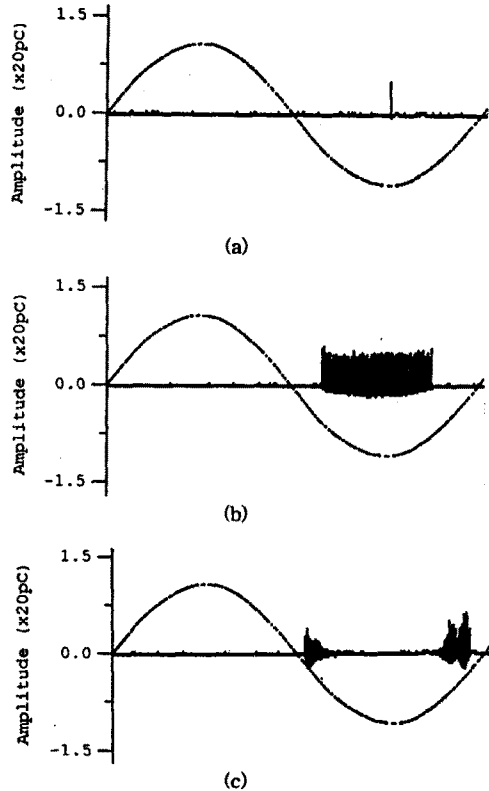
그림 3.4 관측된 PD펄스
