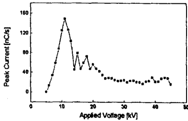
그림 3.2 인가전압-방전 전류의 관계
