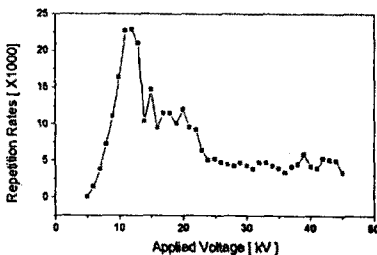
그림 3.3 인가전압-부분방전 발생 빈도수
