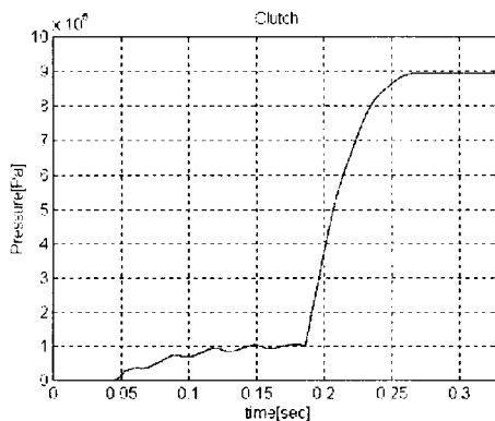
그림 6 시뮬레이션 결과
