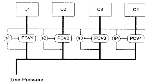
그림 4 전체 유압회로
