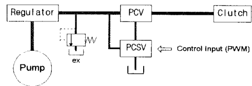
그림 3 직접구동 간접제어 방식의 유압회로
