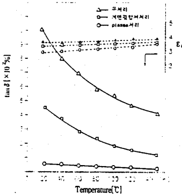
그림 8. 유리섬유 강화 복합재료의 유전 특성
