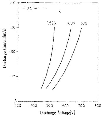
그림 4. 일정 압력하에서 자기변화에 대한 방전전압-특성
