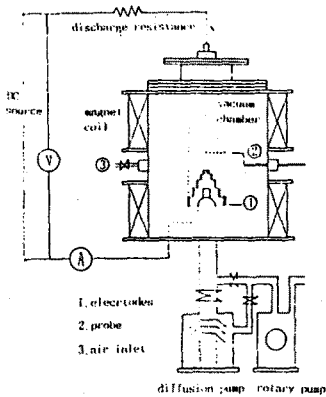
그림 1. 표면처리 장치 개략도
