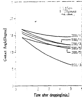
그림 6. 플라즈마 표면처리 조건변화에 따른 접촉각의 변화특성
