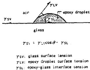
그림 3. 액적의 접촉각
