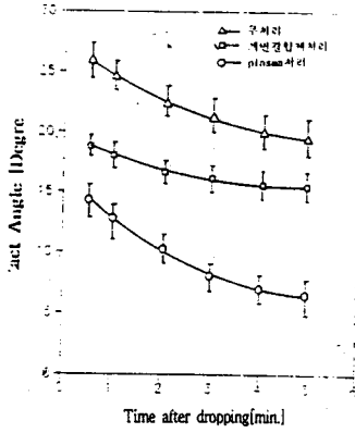
그림 7. 플라즈마, 계면 결합제, 미처리 시료의 접촉각 변화 특성
