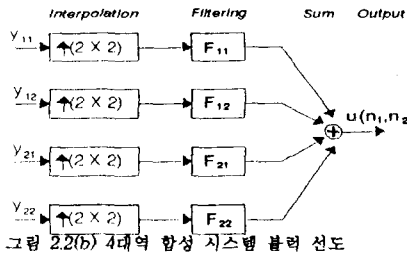
그림 2.2(b) 4대역 합성 시스템 블럭 선도 Fig. 2.2(b) block diagram of 4-band recombination system
