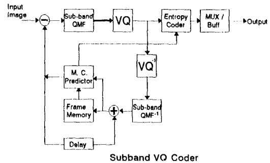
그림 4.2 심장조영상을 위한 Subband-VQ Fig. 4.2 Subband-VQ for angiography
