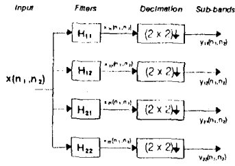
그림 2.2(a) 4대역 분할 시스템 블럭 선도 Fig. 2.2(a) block diagram of 4-band splitting system
