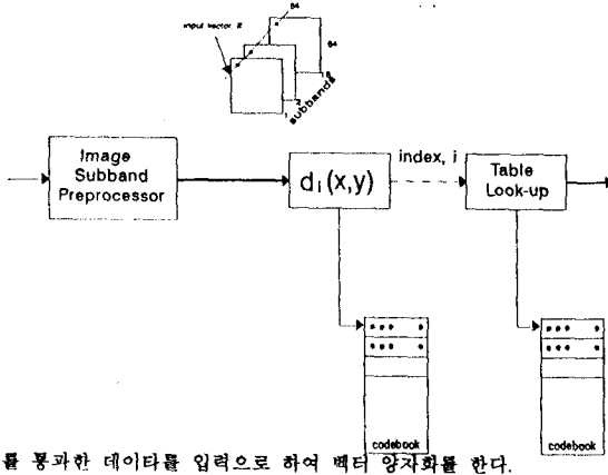
그림 4.1 부대역 벡터 양자화기 Fig.4.1 Subband Vector Quantizer
