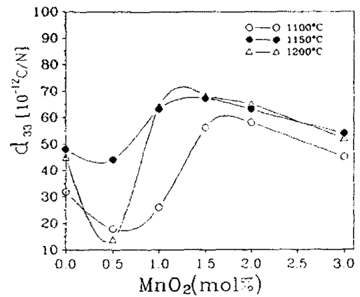
그림 7. MnO_2 첨가량과 소성온도에 따른 압전상수 d_{33} 의 변화
