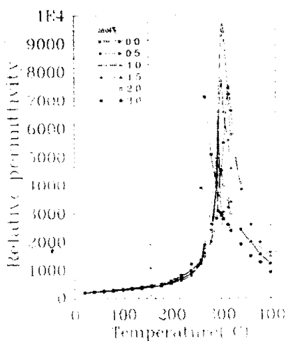
그림 3. MnO 2 첨가량에 따른 비유전율의 온도 의존성 Fig. 3. Temperature dependence of relative permittivity with MnO 2 additive
