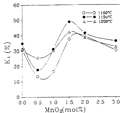
그림 5. MnO 2 첨가량과 소성온도에 따른 전기기계 결합계수 k t 의 변화 Fig. 5. Variation of electromechanical coupling factor k t with MnO 2 additive and sintering temperature
