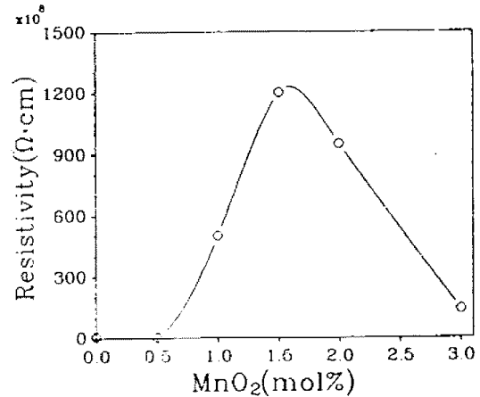
그림 4. MnO 2 첨가량에 따른 저항율 변화 Fig. 4. Variation of resistivity with MnO 2 additive
