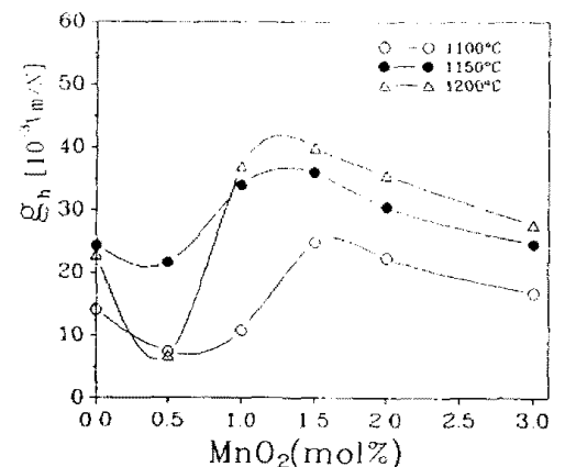
그림 9. MnO_2 첨가량과 소성온도에 따른 압전상수 g_h 의 변화
