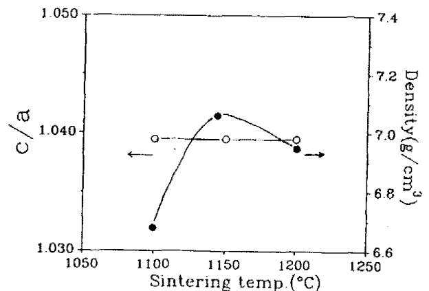
그림 2. 소성온도에 따른 정방성과 밀도 변화 Fig. 2. Variation of tetragonality and density with sintering temperature
