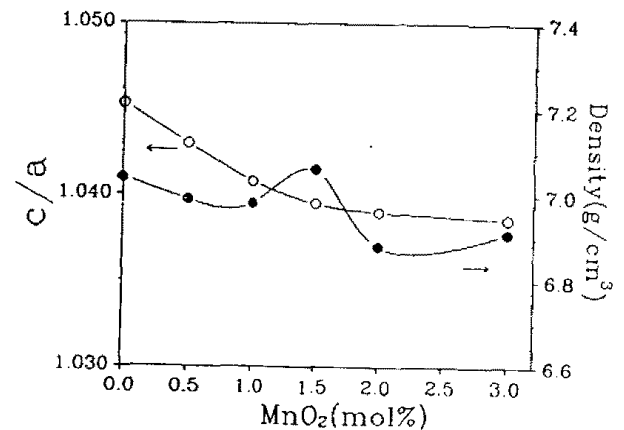
그림 1. \text{MnO}_2 첨가량에 따른 정방성과 밀도 변화 Fig. 1. Variation of tetragonality and density with \text{MnO}_2 additive
