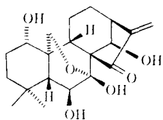
(15) oridonin
