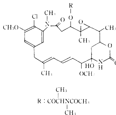
(21) maytansine
