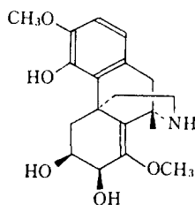
(9) sinococuline
