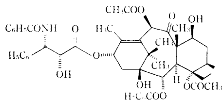
(19) taxol (NSC 125973)
