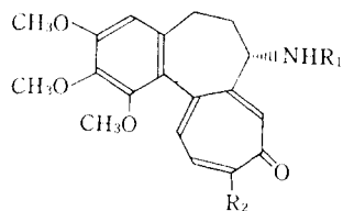
R 1 R 2 (3) COCH 3 OCH 3 (4) CH 3 OCH 3 (5) COCH 3 NH 2
