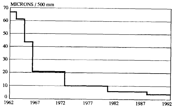
그림 2. 터치 프로브에 의한 측정정도의 개선 추이
