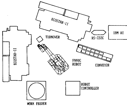
그림 3. 선삭 자동화 셀
