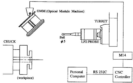
그림 4. 터치 프로브의 설치도
