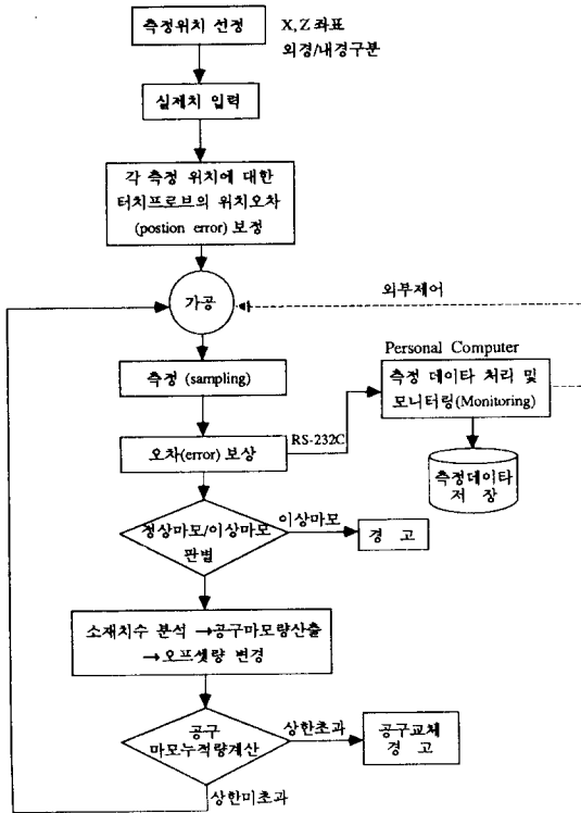
그림 9. 감시 시스템의 흐름도
