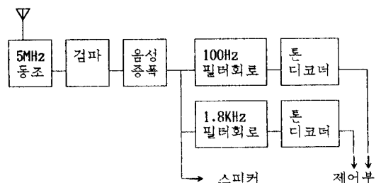
그림 2. 수신부 블록도
