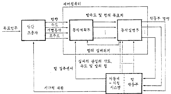
그림 1. 다각 보행로봇의 관리제어 시스템 구조
