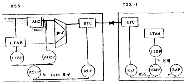
그림 5. 가입자회로 시험 (in-test)
