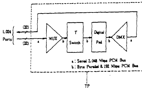
그림 3. 자체로 연결시의 통화로 구성
