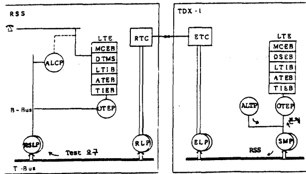
그림 6. 가입자선 시험 (out-test)
