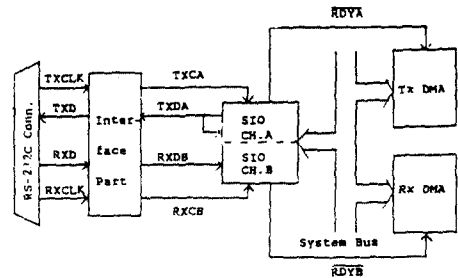
그림 4. 데이터링크 인터페이스 외도
