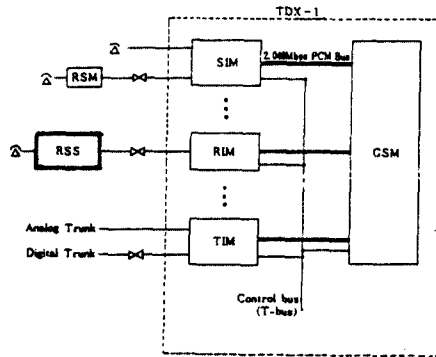
그림 1. TDX-1 시스템 구조
